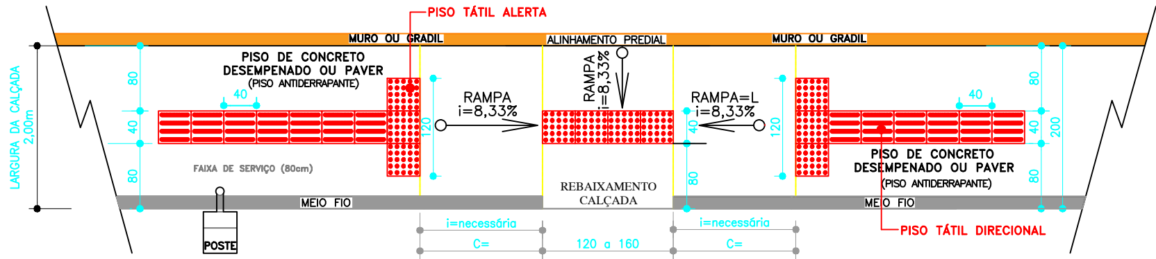
DESENHO III Planta Baixa Calçada Rebaixamento p/ Cadeirante
