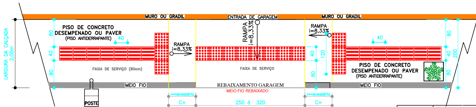
DESENHO IV Planta Baixa Calçada Rebaixamento entrada de Garagem
